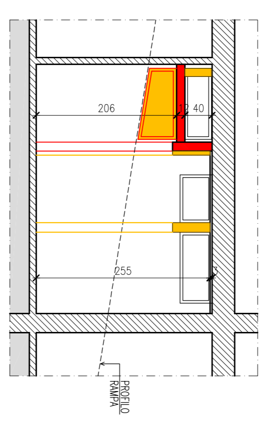
SEZIONE A-A
